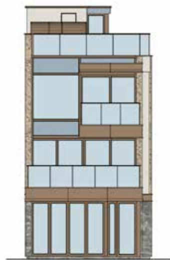
ELEVATION PLAN 1 立面圖 1
