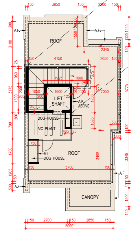
Upper Roof Plan 上層天台平面圖
